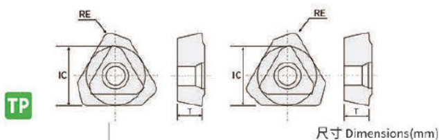
尺寸 Dimensions(mm)
