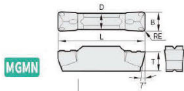
尺寸 Dimensions(mm)
