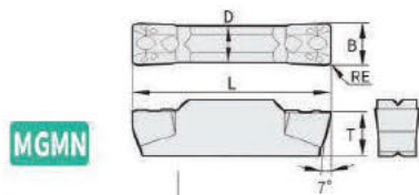
尺寸 Dimensions(mm)
