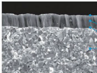
PVD涂层横截面图
